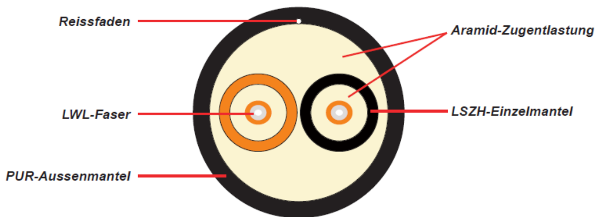
Bild/Pic. 1 Skizze: Abisolirtes Kabel mit Querschnitt und Beschreibung / 1 Sketch: Stripped cable with cross-section and description
